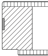
Einleimer sichtbar, Brandschutzquellstreifen sichtbar
